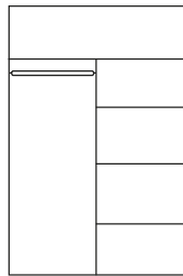
ARMOIRE BRUARM 20 1/2 penderie, 1/2 lingère, 2 portes Larg. 126 x Haut. 195 x Prof. 57
